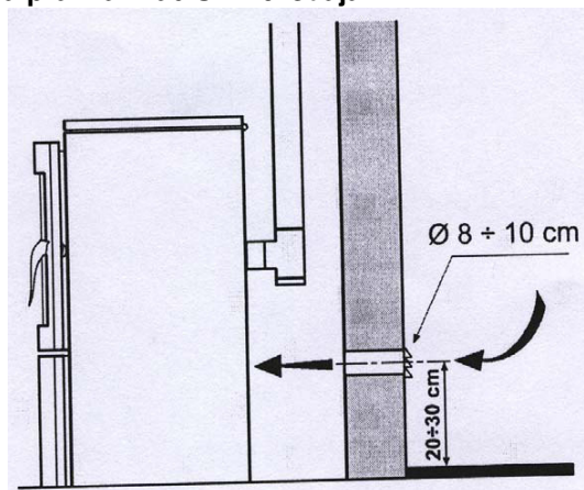
Slika 8. Minimalna rastojanja za postavljanje ventilacione rešetke
